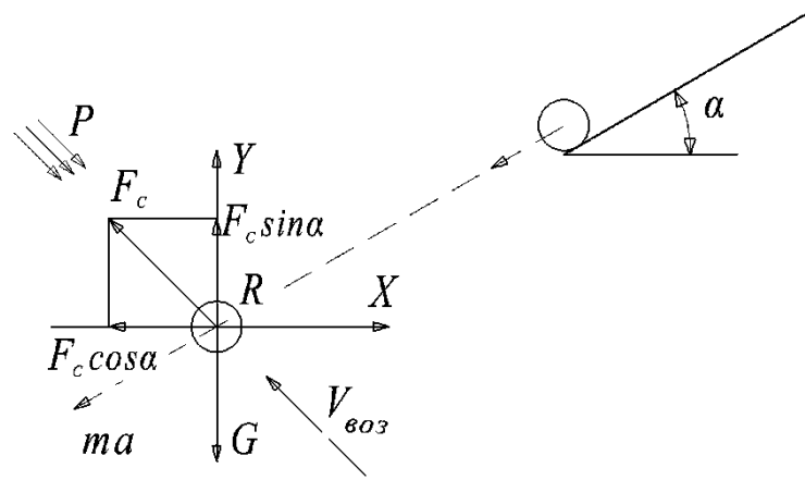
Рисунок – 6. Схема сил, действующих на тело при спуске с наклонного лотка
