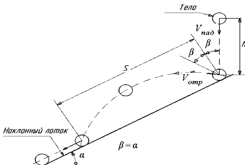
Рисунок - 2 Схема падения, отскока и скольжения тела.
